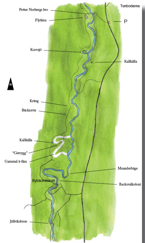
Illustration Lennart Vessberg, ur Mjällådalens geologi
